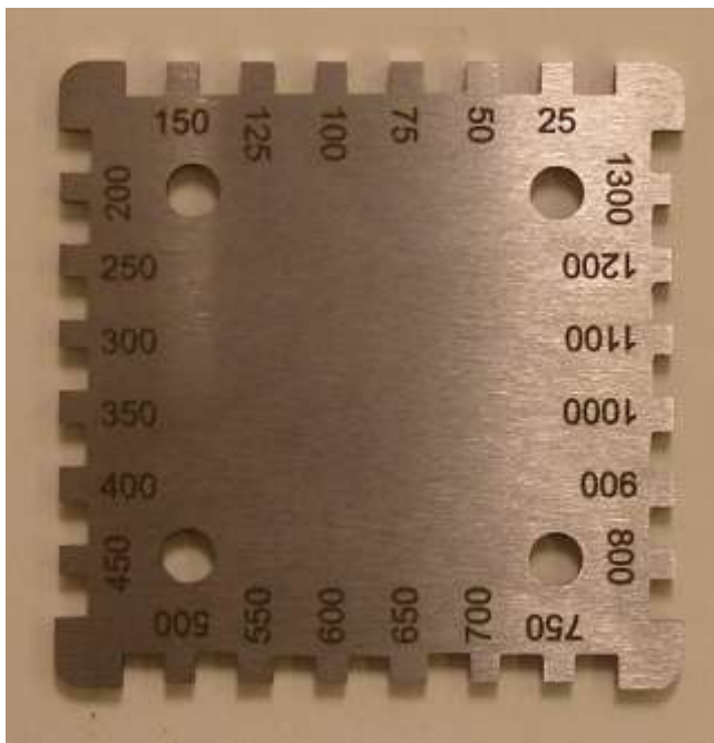
Рис. 1 Измерительная гребенка для определения толщины свеженанесенной краски.
