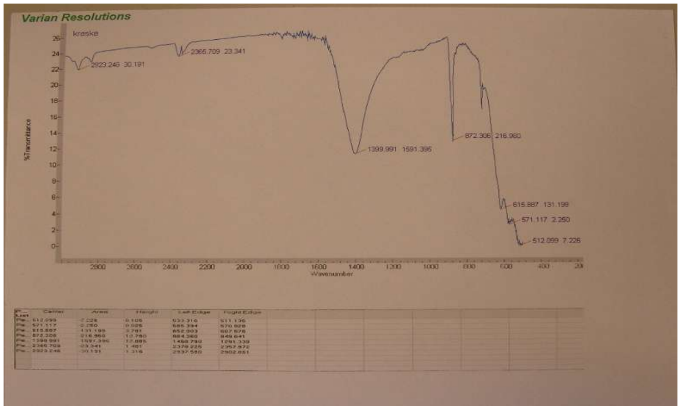
Рис.1 Инфракрасный спектр краски для дорожной разметки.
